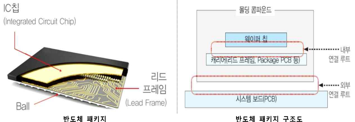
[그림 9] 반도체 패키지 구조도
