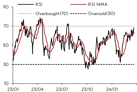
코스닥 RSI
