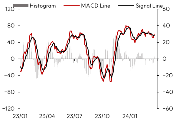
S&P 500 MACD
