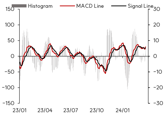
코스피 MACD
