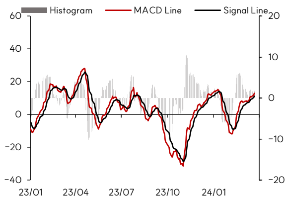
코스닥 MACD
