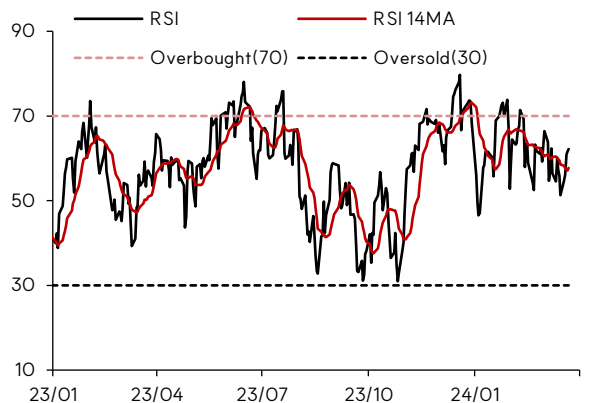
나스닥 RSI
