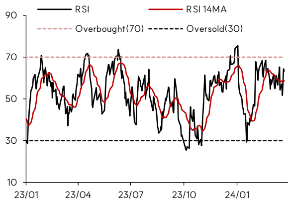
코스피 RSI
